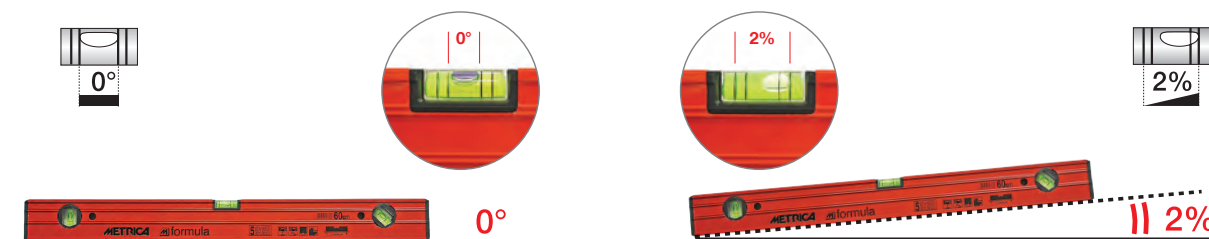
Zentrallibelle mit 4 Streifen: für die 0°-Anzeige (Innenstreifen) oder für 2%-Neigung (Außenstreifen)
