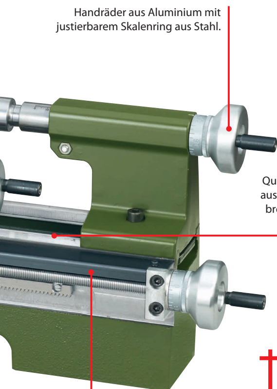
Verkleidete Leitspindel mit Trapezgewinde (12 x 1,5).
